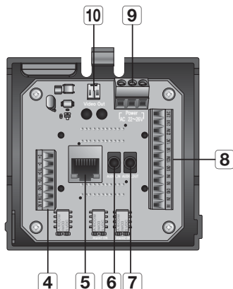
Widok podstawy instalacyjnej wewnątrz
